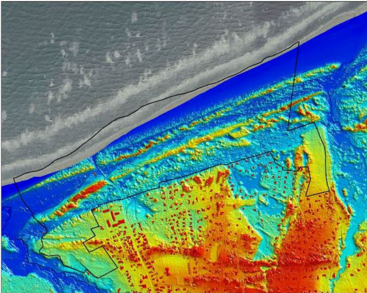
Figur 5-1 Kort som viser de topografiske forhold i fredningen (sort afgrænsning). (Baggrundskort DTM 2015).
